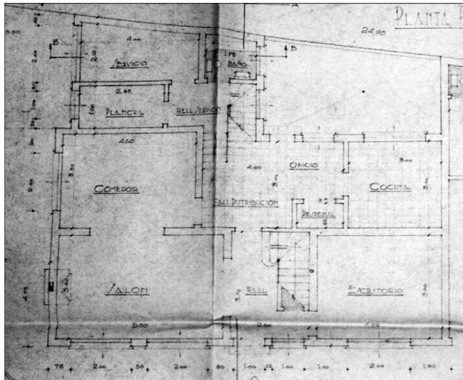
PLANTA PRIMERO PISO
